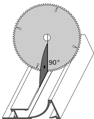
Tarcza do cięcia aluminium Aluminium cutting saw blade Sägeblatt für Aluminium Пильный диск по алюминию
